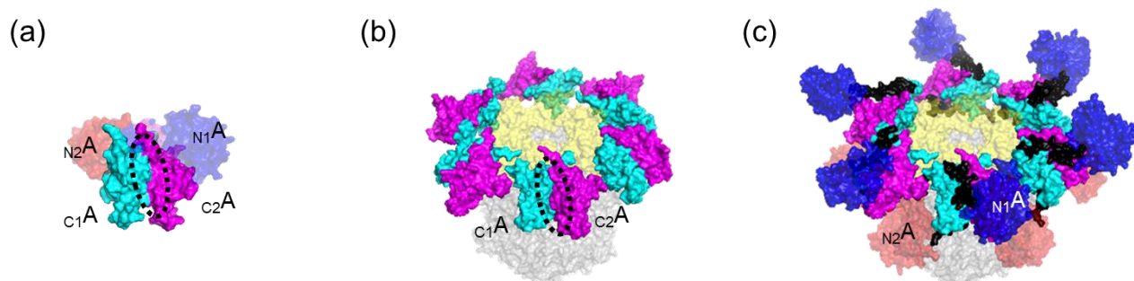
図 2： ABC 三者複合体上の KaiA の立体配座。KaiA は 2 量体であり、各単量体は 2 つのドメインを持っています。図では、1 つの KaiA の N 末端側ドメインと C 末端側ドメインをそれぞれ N_1A (青)と C_1A (水)、もう一つの KaiA の N 末端側ドメインを N_2A (赤)と C 末端側ドメインを C_2A (紫)として、色で塗り分けて表しています。 (a) KaiA2 量体上の KaiC との相互作用界面（黒点線枠）を示しています。 (b) 低温電子顕微鏡により解かれた ABC 複合体の構造です。KaiA2 量体の N 末端側ドメインである N_1A (青)と N_2A (赤)が観測されていません。そのため、(a)で示した相互作用界面が外部に暴露しています。 (c) ABC 複合体の全長構造です。 N_1A と C_1A をつなぐループを黒で示していますが、特に今回解明した N_1A とループの配置が、相互作用面が暴露することを防いでいる様子を捉えています。
